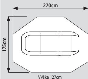
Vnitřní rozměry podlahy
