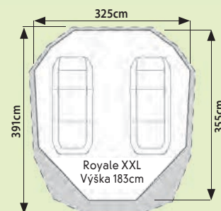
Vnitřní rozměry podlahy
